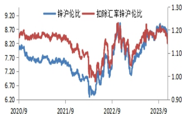
图2：锌沪伦比值
