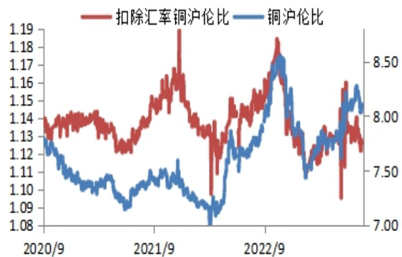
图4：铜沪伦比值
