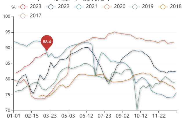
2023-03-17,247家钢厂产能利用率
