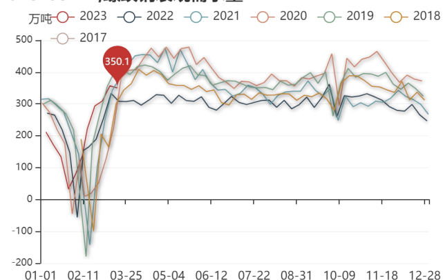
2023-03-17,螺纹钢表观需求量
