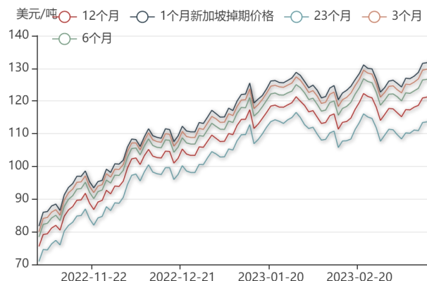
2023-03-15,新加坡掉期价格
