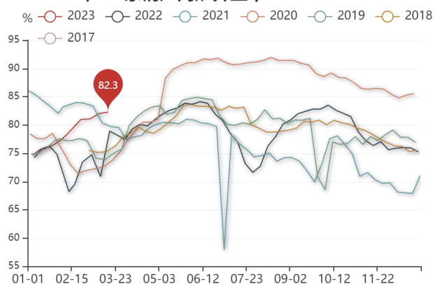
2023-03-17,247家钢厂高炉开工率
