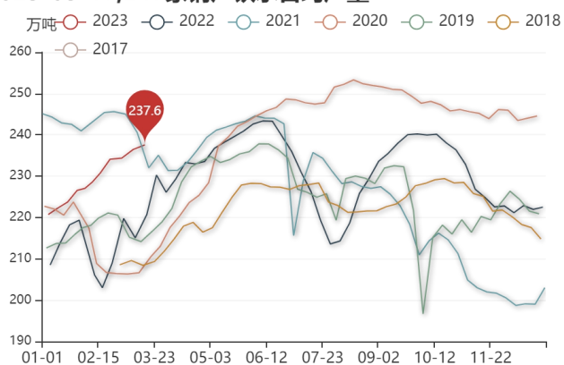
2023-03-17,247家钢厂铁水日均产量
