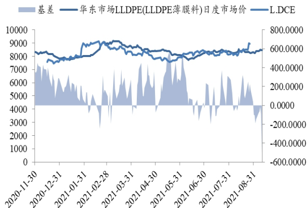
图1: L基差(元/吨)
