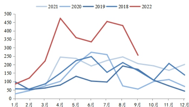
图9: PE检修损失量(千吨)
